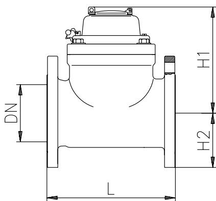
Dimensiones WPH-N
