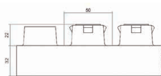
Detalle del perfil (cotas en mm)
