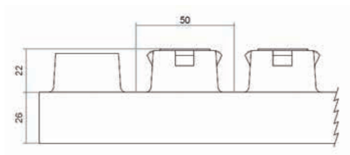
Detalle del perfil (cotas en mm)
