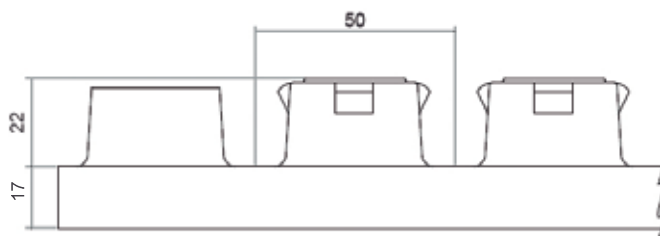
Detalle del perfil (cotas en mm)
