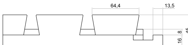
Detalle del perfil (cotas en mm)
