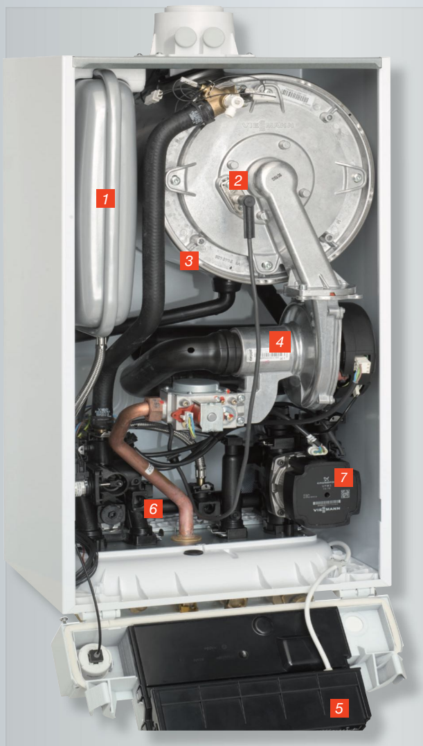
Caldera mixta con producción instantánea de A.C.S.
