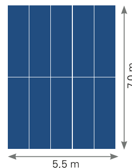
Ejemplo de disposición de módulos para pack FV XL , superficie necesaria 5,5 x 7,0 m
