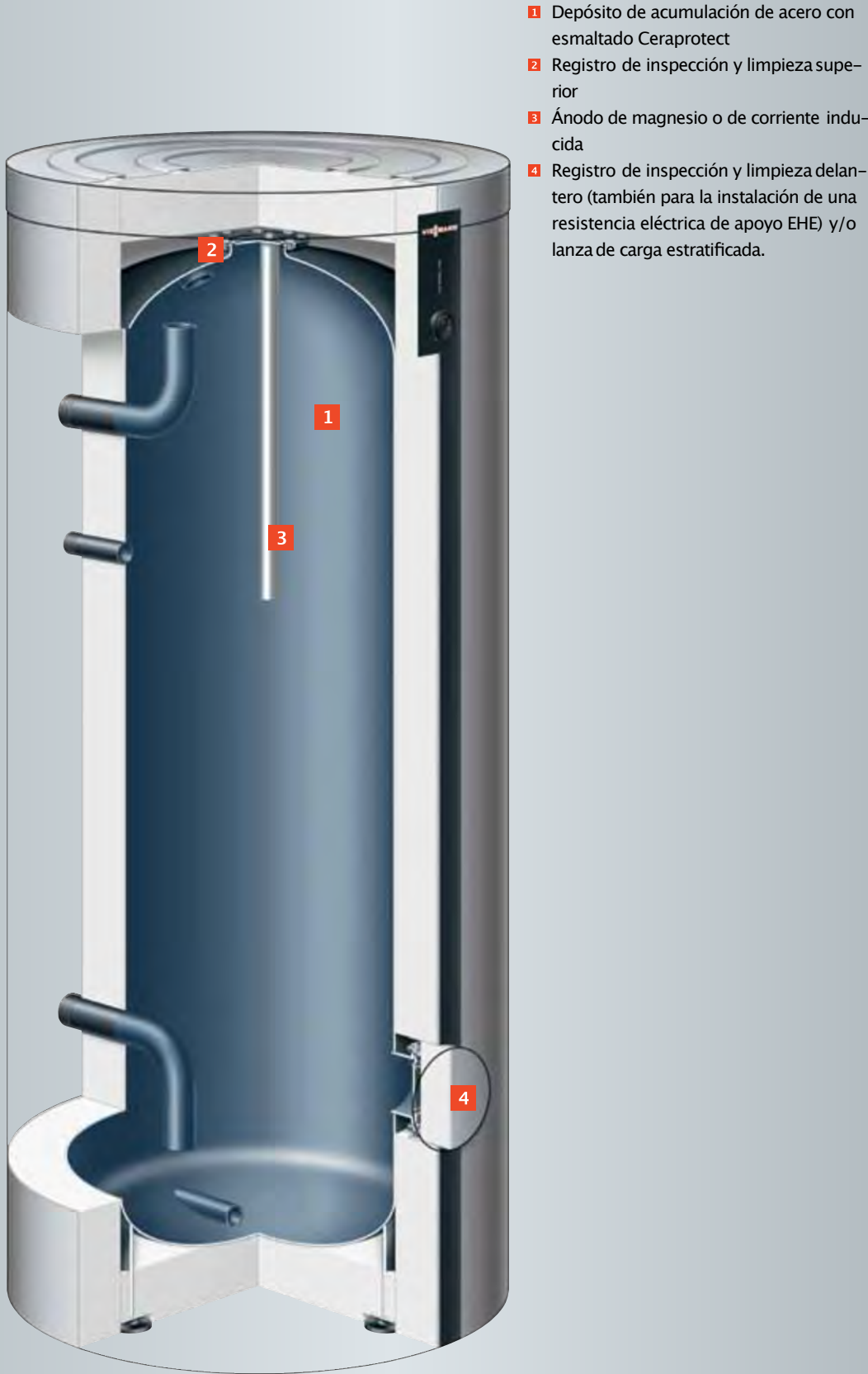
Vitocell 100-L (Modelo CVL, volumen de 500 litros)
