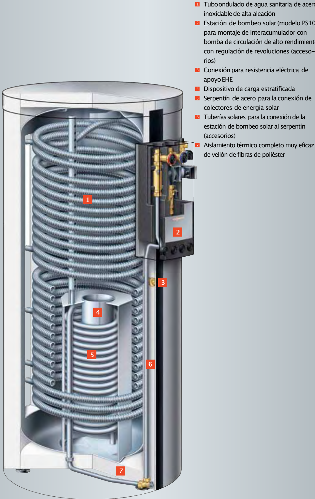
Vitocell 360-M con Solar-Divicon (accesorios) (modeloSVSA)
