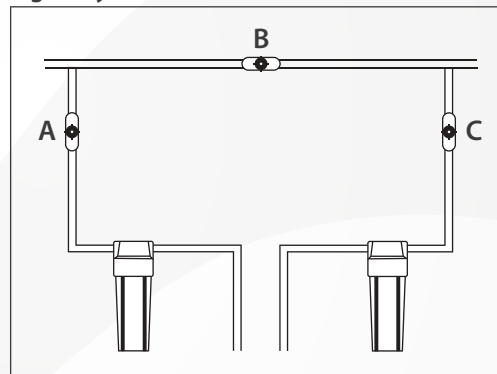
Fig. 2: By-Pass - Fontanería
